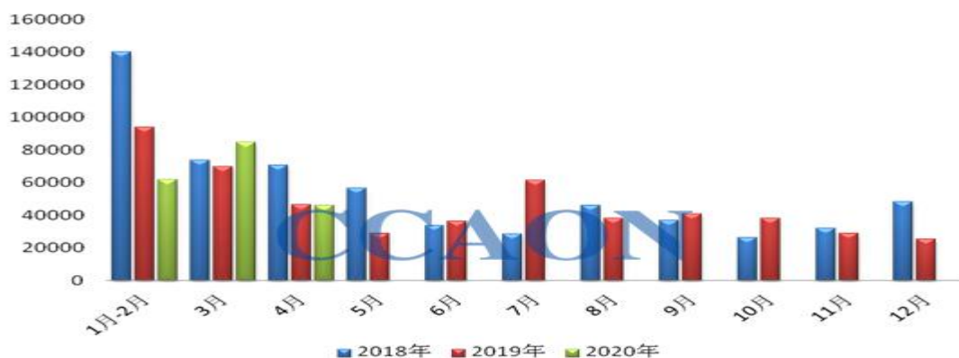
2018-2020 年我国 PVC 出口量（单位：吨）
